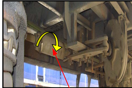
Slack adjuster
